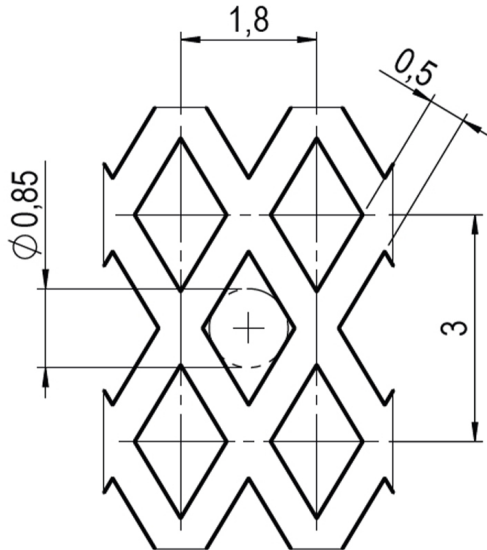
SZITA JELLEMZŐI átömlési keresztmetszet = 43%
